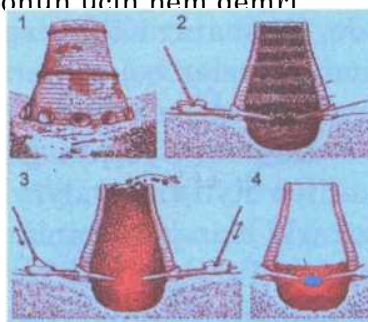
Demir eredilýän küräniň görnüşi
